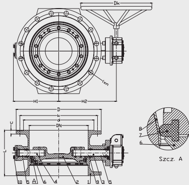
Valvola a farfalla doppio eccentrico flangiata
