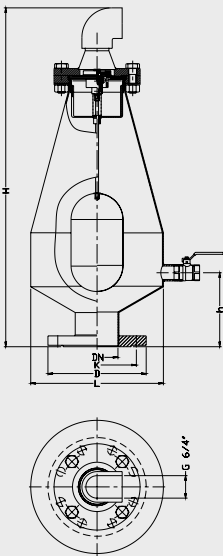
Collegamento a flangia.
