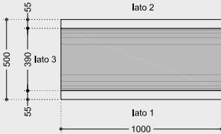
Caditoia leggera
