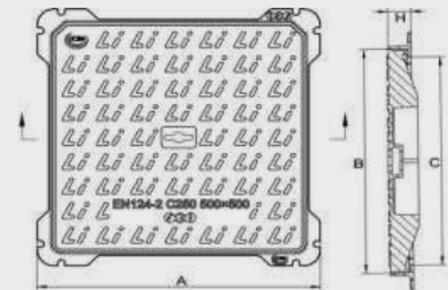
Chiusino con telaio e coperchio rettangolari per derivazioni fibra ottica. Classe C250
