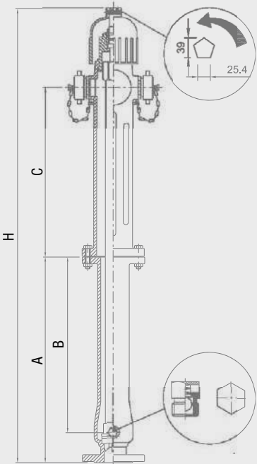
Idrante sopra suolo in ghisa - 2 attacchi
