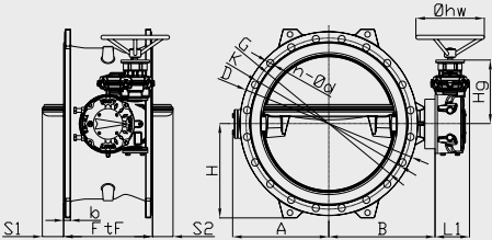
Valvola a farfalla doppio eccentrico biflangiata
